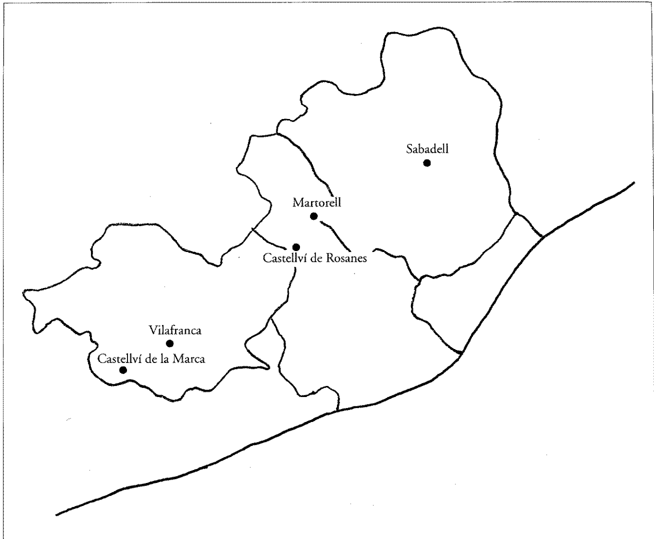
IL·LUSTRACIÓ 1. Esquema que mostra l'emplaçament dels dominis més meridionals de les baronies dels Montcada.
