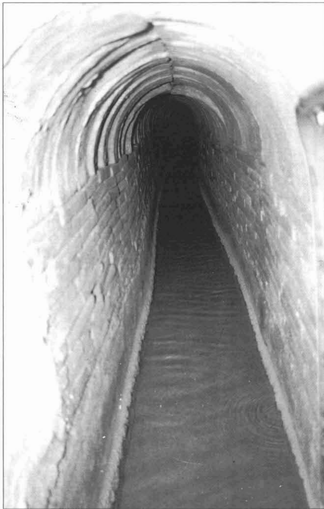
FOTOGRAFIA 4. Interior de la mina d'aigua de Ribatallada. (Foto: Joan Pérez / Col·lecció CASSA).
