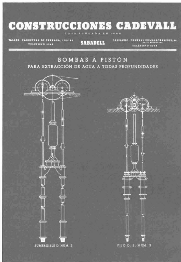
IL·LUSTRACIÓ 2. Esquema de dues bombes de pistó utilitzades per a l'extracció d'aigües subterrànies. Reproducció extreta d'un catàleg de Construccions Cadevall. (Foto: Col·lecció CASSA).
