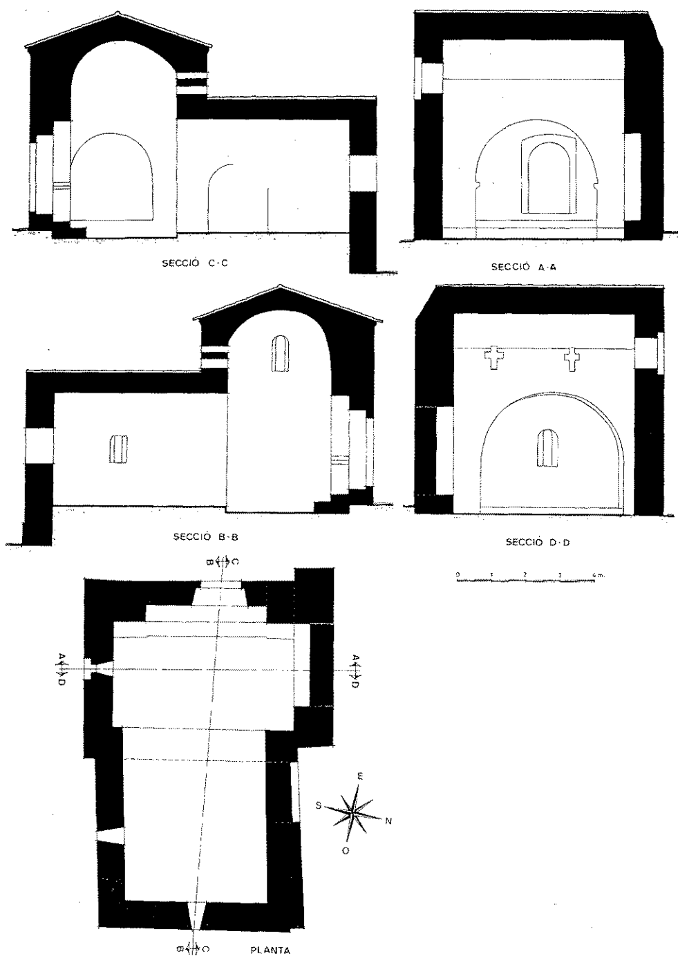
Figura 4 A. Plànols de Sant Nicolau, aixecats durant aquests treballs.
