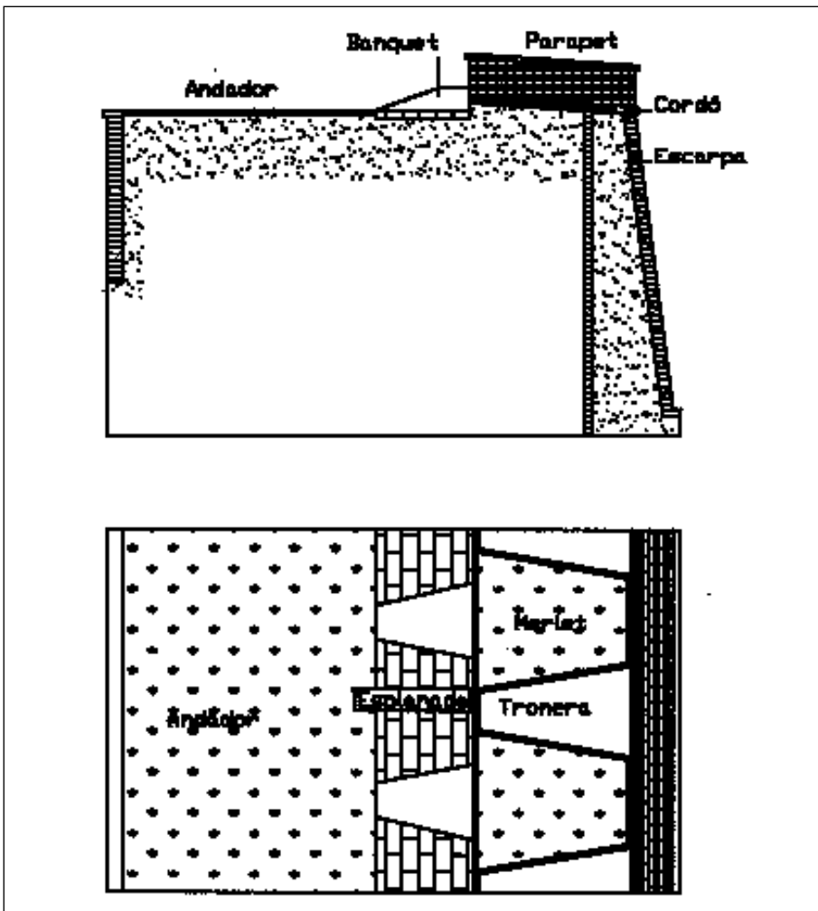
Figura 2. Esquema del terraplè. Alçat i planta.
