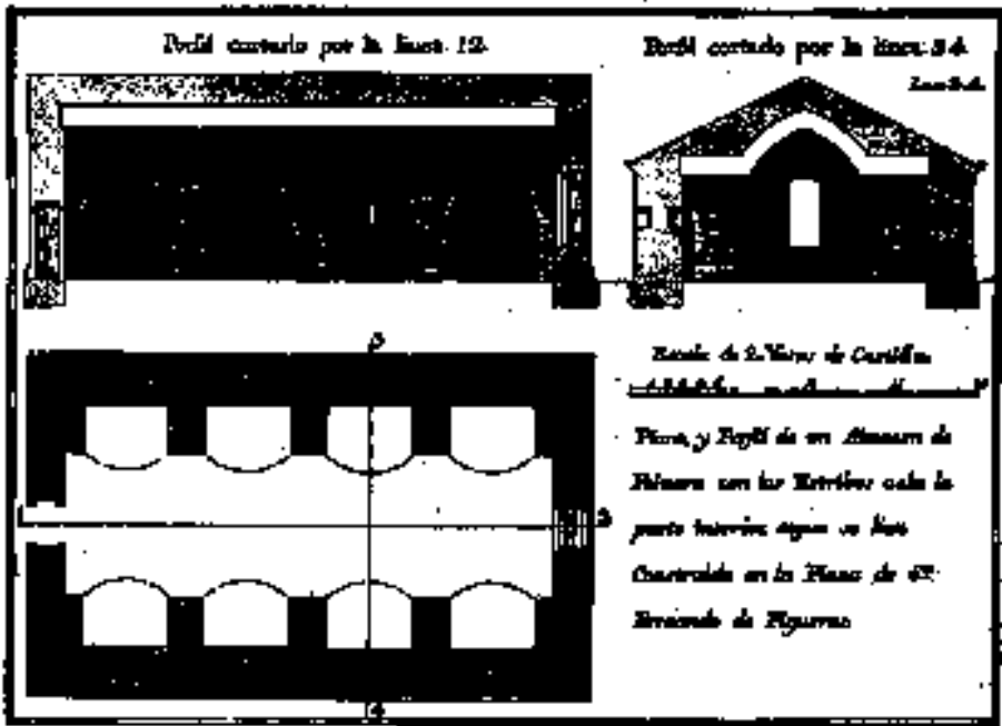
Figura 3. Polvorí de Sant Jaume. Làmina del llibre "Tratado de fortificación o arte de construir edificios militares y civiles". M. Sánchez Taramas. Barcelona, 1769.
