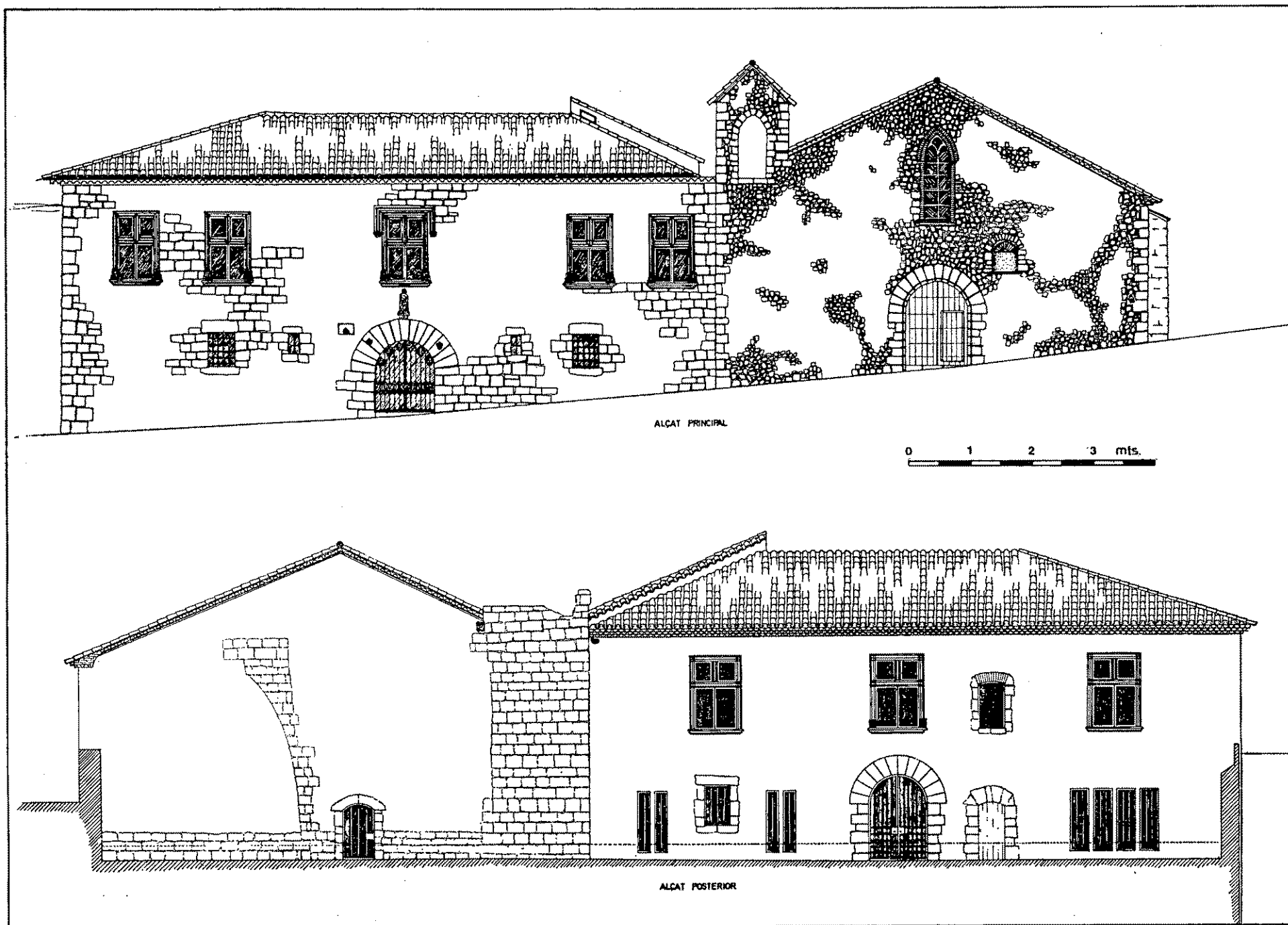
Lám. I. Hospital de Santa Magdalena. Alçat principal i alçat posterior.
