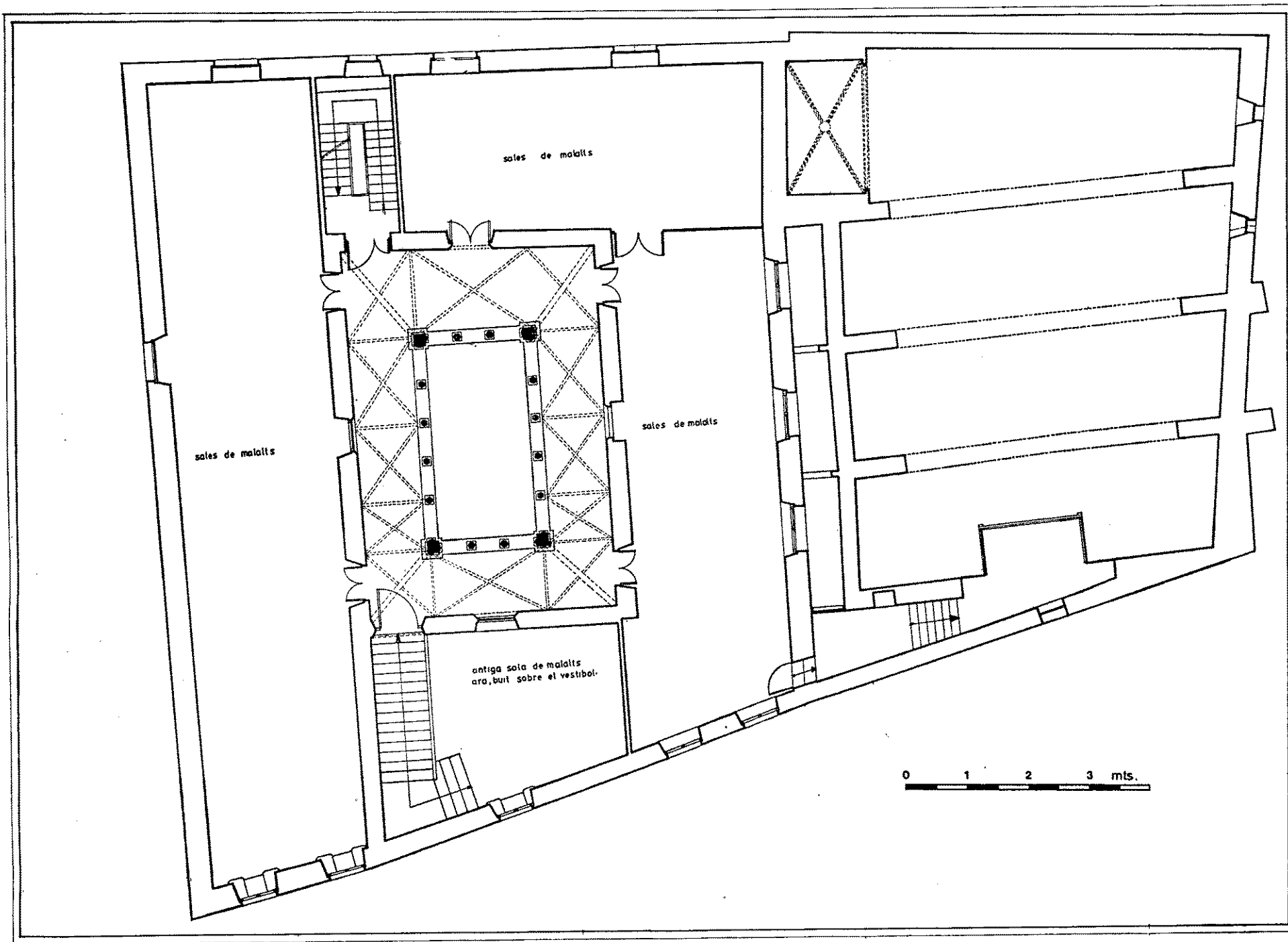
Làm. III. Hospital de Santa Magdalena. Planta del primer pis.
