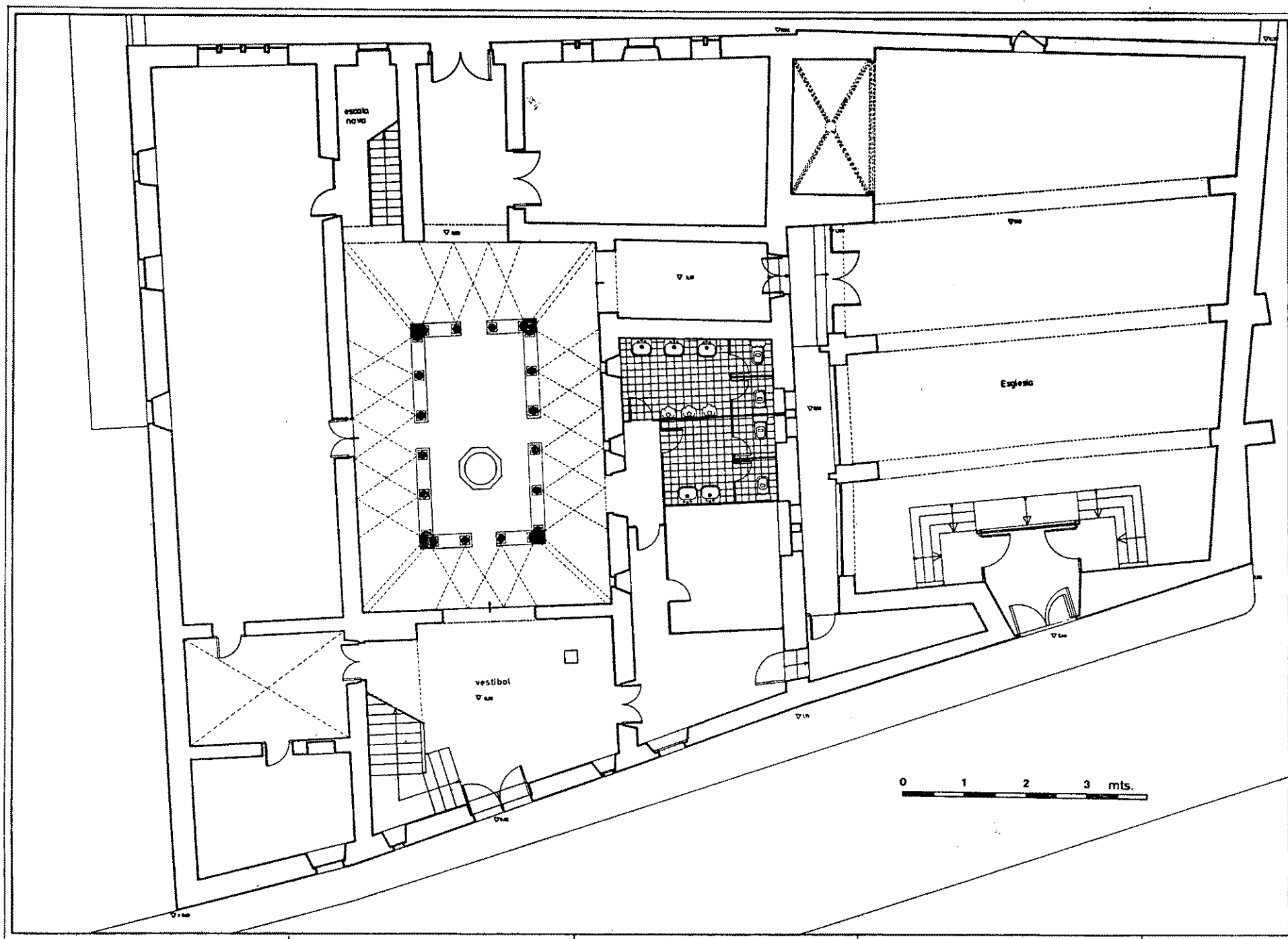
Lâm. II. Hospital de Santa Magdalena. Planta baixa.
