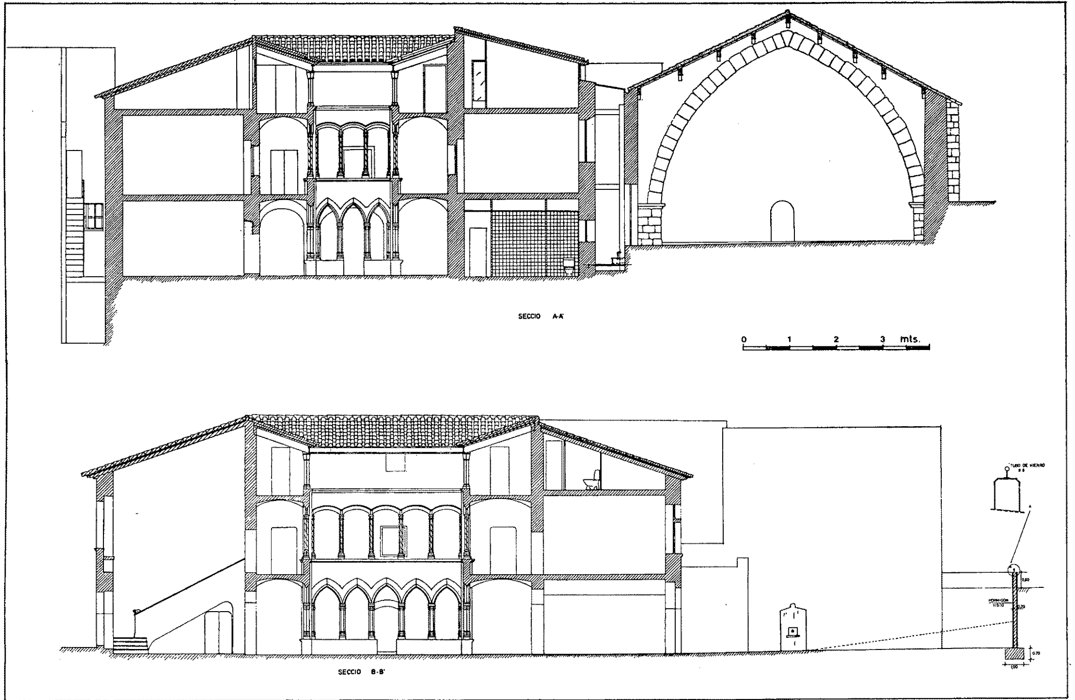
Làm. IV. Hospital de Santa Magdalena. Seccions longitudinal i transversal.
