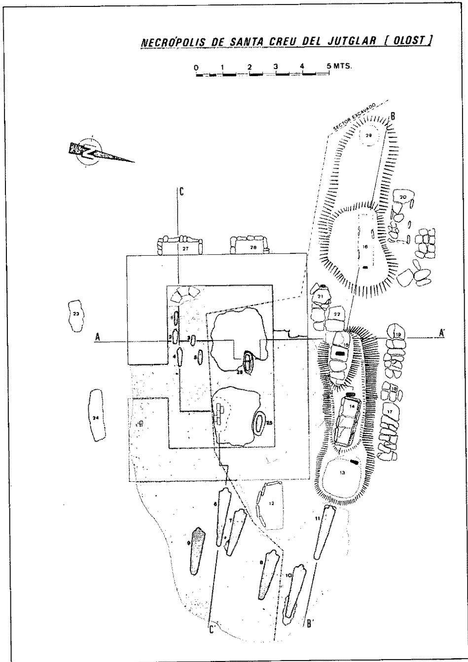
FIG. 3. Plànol general del jaciment, completat amb les dades proporcionades pels Diaris d'Excavació.
