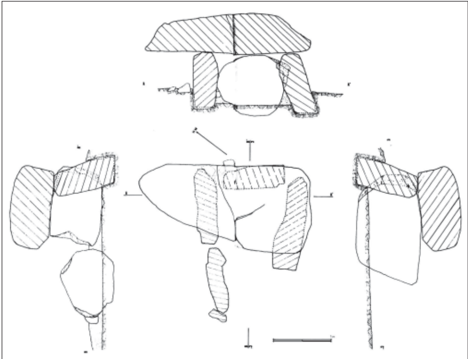
Planta i seccions del dolmen de la Roca d'En Toni (CASTELLS i VILARDELL 1983: 50-51).
