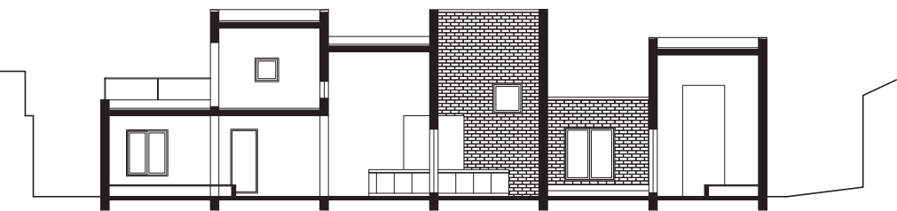
Secció A Section A
