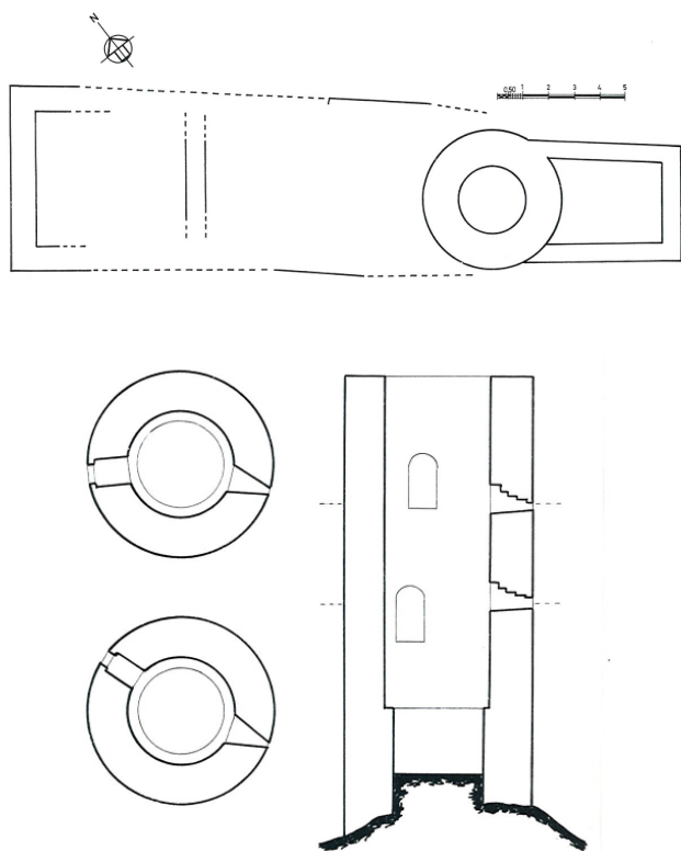
Figura 4. Planta del castell de la Baronia de Sant Oïsmo, i de la seva torre circular (J.Bolós / Enciclopèdia Catalana)
