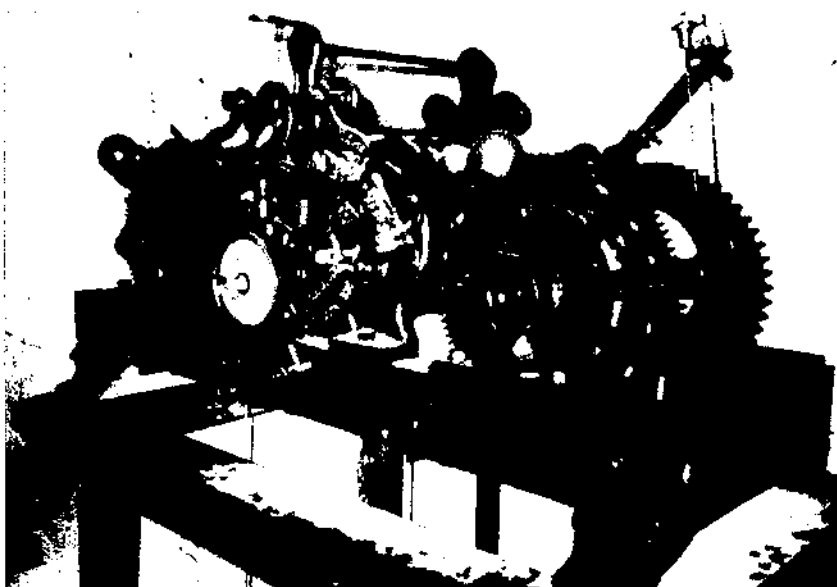
Maquinària del rellotge del campanar, construït per Josep Besses, de Tarragona, a finals del segle XIX, i que encara funciona.
