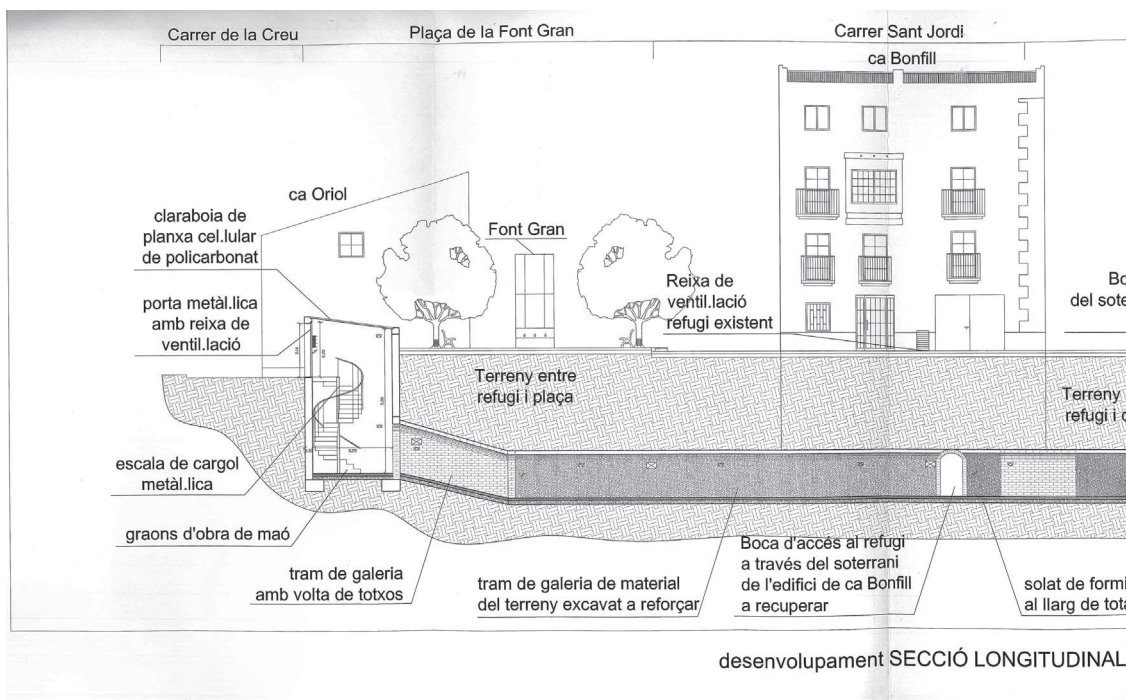
Fig. 6. Plànol topogràfic del traçat del refugi de la Font Gran. Elaborat per Agustí Piñol. Ajuntament de Benissanet.
