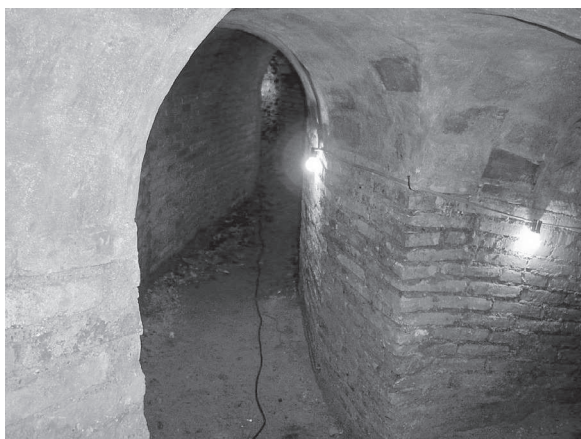
Fig. 3. Tram d'obra del final del passadís dret a l'altura de la Font Gran.
