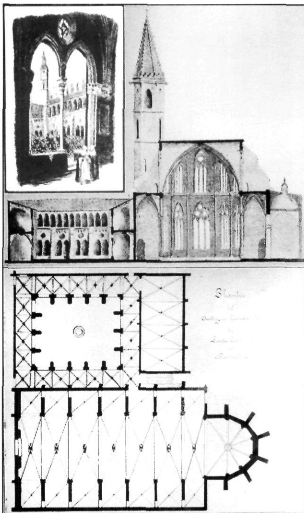
Planta i alçat del desaparegut convent de Santa Caterina de Barcelona.
