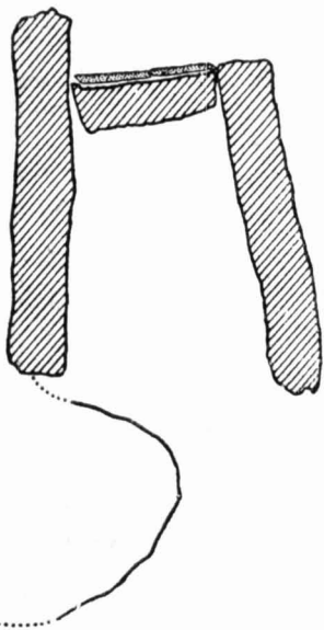
Fig. 4. — Planta del megalito menor de Biescas. Escala 1 : 20
