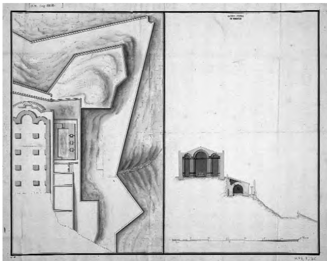
Figura 5: [Proyecto de un almacén de pólvora]. [1718] Arxiu: Archivo General de Simancas (Simancas-Valladolid)
