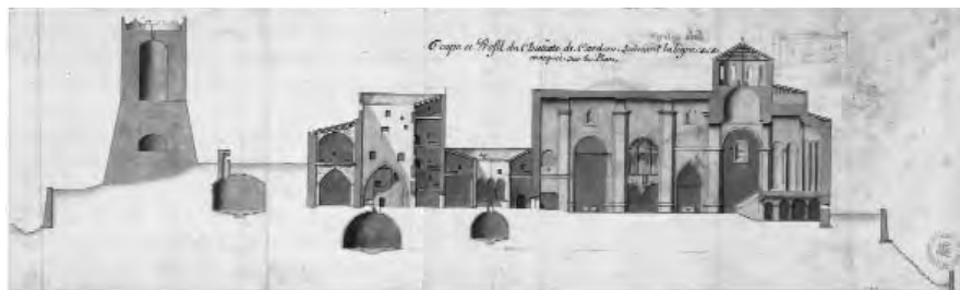
Figura 10: Coupe et profil du Chateau de Cardone suivant la ligne zz, marque sur le plan. [1721] Arxiu: Centro Geográfico del Ejercito. Archivo Cartográfico y de Estudios Geográficos (Madrid)
