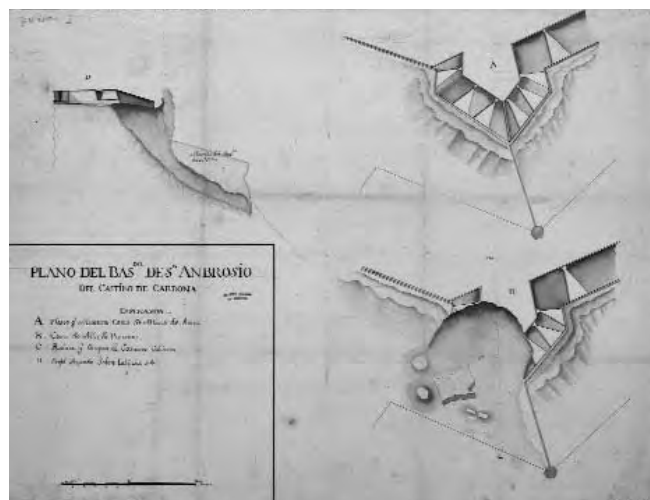
Figura 11: Plano del bastión de San Ambrosio del castillo de Cardona. [1721] Arxiu: Archivo General de Simancas (Simancas-Valladolid)
