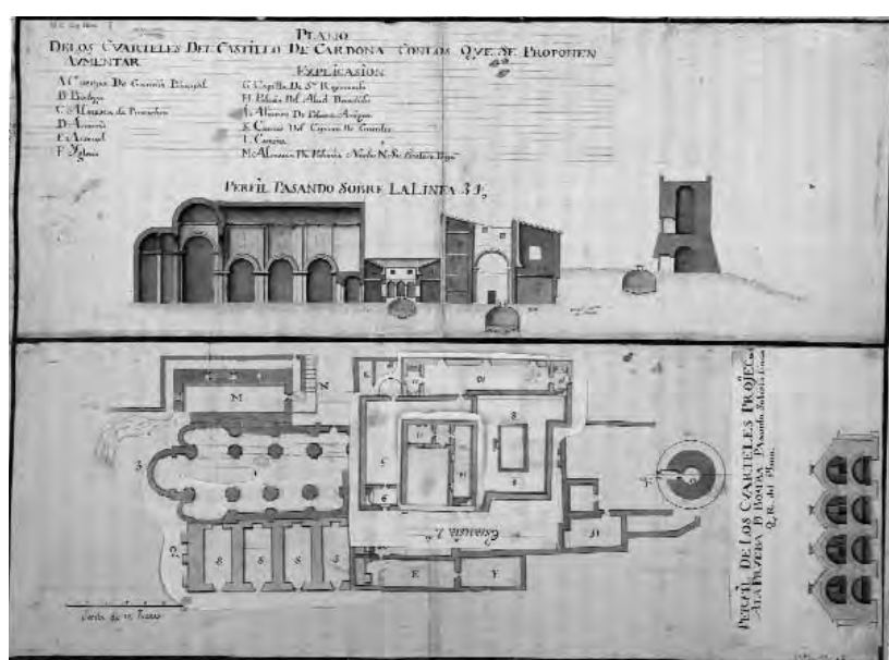
Figura 15: Plano de los curteles del castillo de Cardona con los que se proponen aumentar. [1718] Arxiu: Archivo General de Simancas (Simancas-Valladolid)
