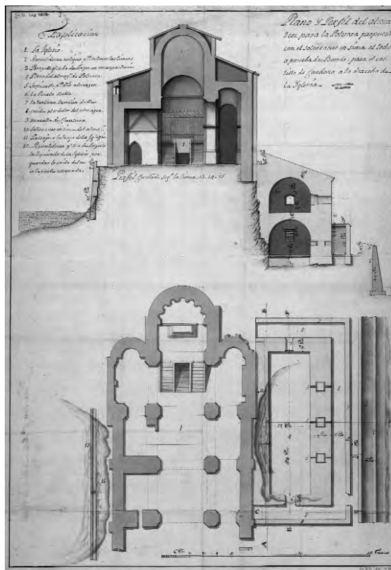
Figura 7: Plano y perfil del almacén para la pólvora propuesto con el soterraneo encima, el todo a prueba de bomba, para el castillo de Cardona a la derecha de la iglesia . [1718] Arxiu: Archivo General de Simancas (Simancas-Valladolid)
