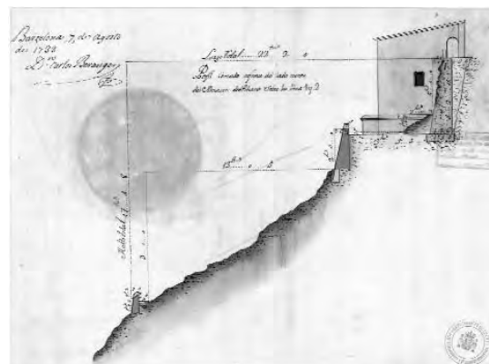
Figura 14: Perfil cortado enfrente del lado menor del Almacen de Pólvara Sobre la línea 1 y 2. 1733 Arxiu: Centro Geográfico del Ejército. Archivo Cartográfico y de Estudios Geográficos
