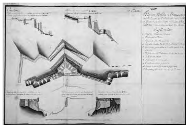
Figura 12: Planos, perfiles y elevaciones del baluarte de San Ambrosio en el castillo de Cardona, en donde está señalado el baluarte existente, y como conviene hacer su restablecimiento. 1721 Arxiu: Archivo General de Simancas (Simancas-Valladolid)
