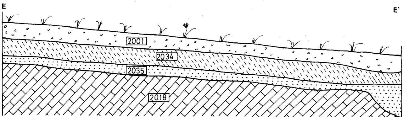
Fig. 3.- Puig Rodon, Sector 2. Seccions D/D' (est-oest) i E/E' (nord-sud).
