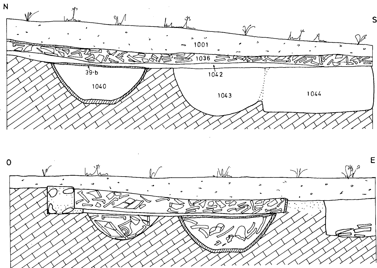
Fig. 19.- Puig Rodon, Sector 1. Seccions nord/sud i est/oest de l'Habitació dels dolia (vegeu planta a CASAS J. (1986), p. 19, fig. 2).
