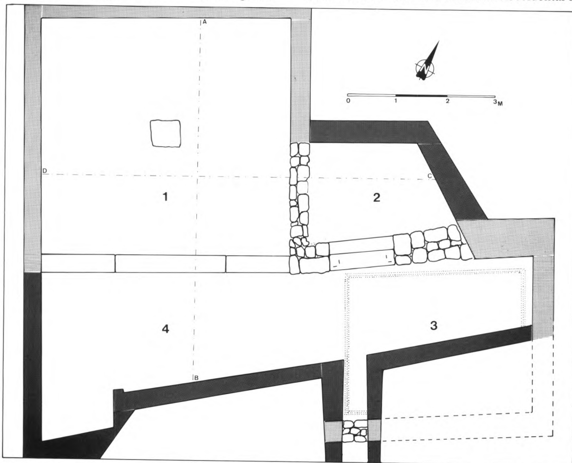
Fig. 4.— Planta de les estructures conservades de la vil·la romana de Can Martí. Amb trama de punts, els murs romans damunt dels quals s'ha refet la construcció antiga. Amb trama fosca, els murs de contenció contemporanis que delimiten les restes visibles.
