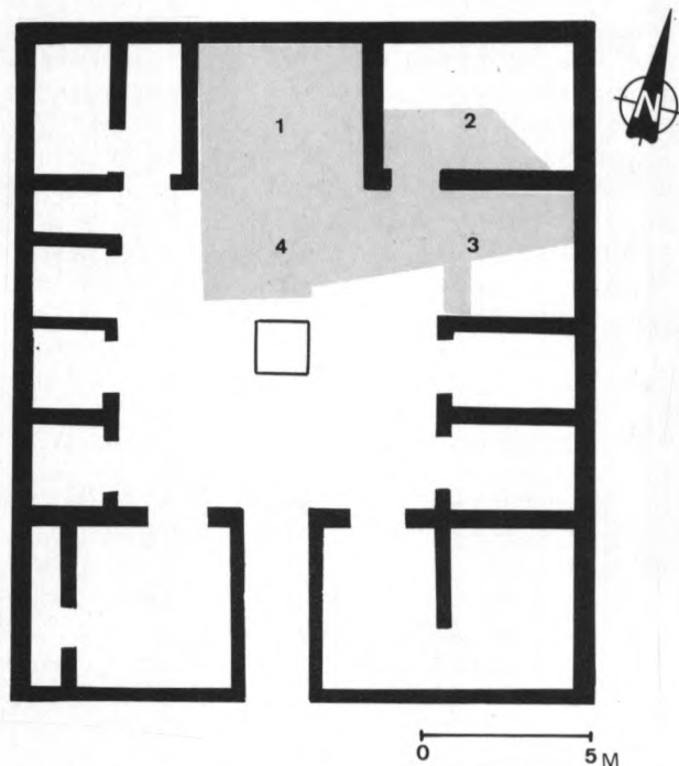
Fig. 15.- Esquema clàssic de la pars urbana d'una vil·la romana. Amb trama i numerats, els àmbits identificats segons les estructures conservades en la vil·la de Can Martí.
