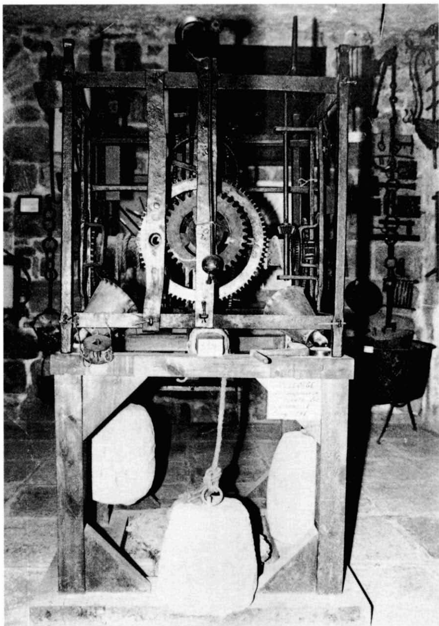
Fig. 3. Rellotge de pesos del campanar de ca l'Isanta o torre de les hores de Solsona. Datat l'any 1795 [Foto: Conxita Flores].
